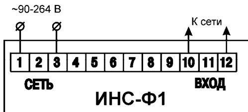
Рисунок Б.1 – Схема подключения прибора ИНС-Ф1.х.ЩЗ
