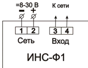
Рисунок Б.2 – Схема подключения прибора ИНС-Ф1.х.Щ9
