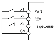
Рисунок 14 – схема подключения закрепленных входов в трехпроводном режиме
