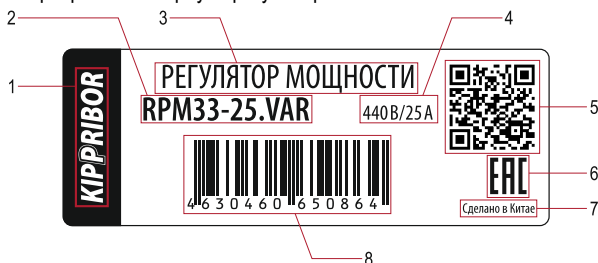
Рисунок 2 – Заводская этикетка регуляторов RPM33
