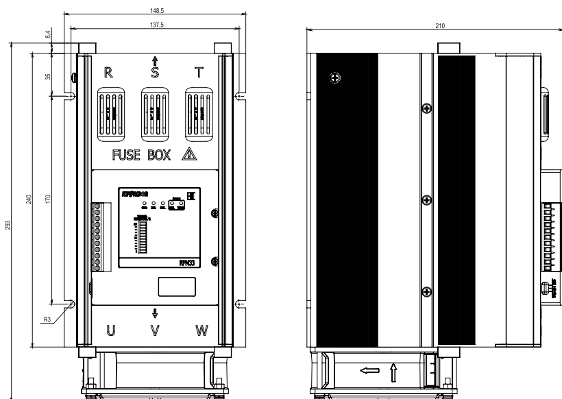
Рисунок 6 – Габаритные размеры RPM33-125.VAR, RPM33-150.VAR, RPM33-200.VAR
